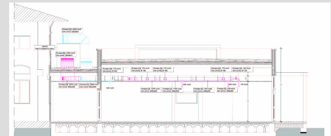
IMPIANTO MECCANICO - VENTILAZIONE MECCANICA
