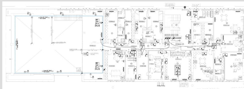
PIANO PRIMO IMPIANTO ELETTRICO
