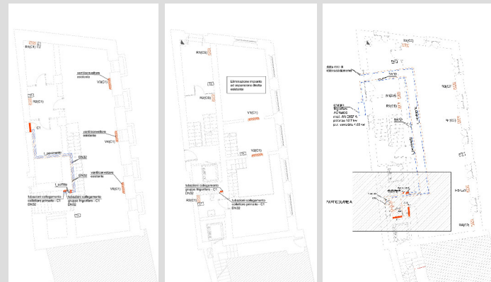
IMPIANTO DI RISCALDAMENTO PIANO INTERRATO TERRA E PRIMO
