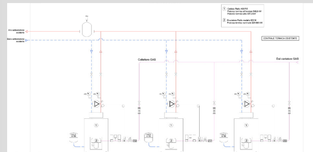
SCHEMA DI CENTRALE TERMICA STATO DI FATTO
