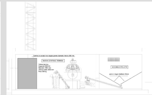
SEZIONE CENTRALE TERMICA
