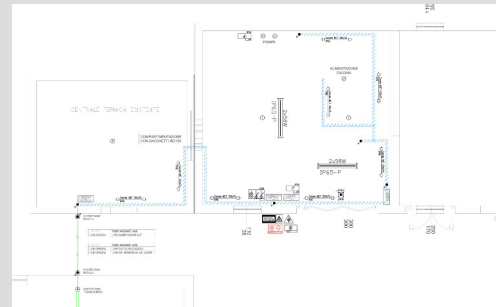
IMPIANTO ELETTRICO
