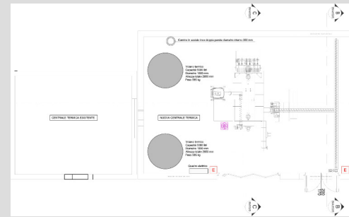
PIANTA CENTRALE TERMICA
