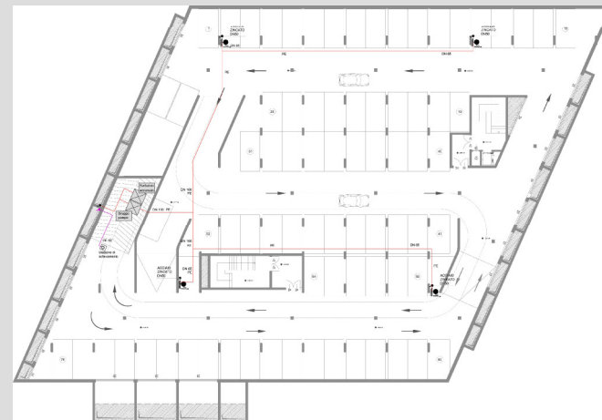
IMPIANTO MECCANICO
